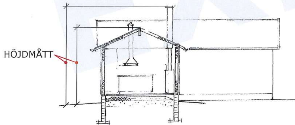
SEKTION TILLBYGGNAD
